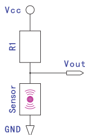
基本电路
