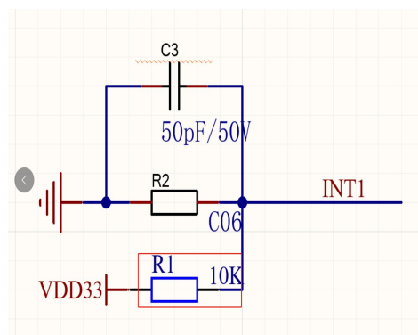
滤波电路
