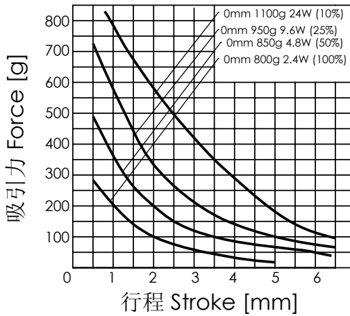
行程 / 吸引力 Stroke and Force
