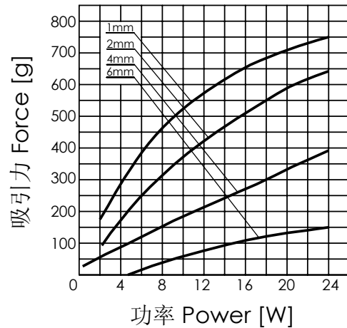
功率 / 吸引力 Power and Force
