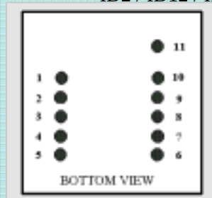
ID2 / ID12 / ID20 PIN-OUT
