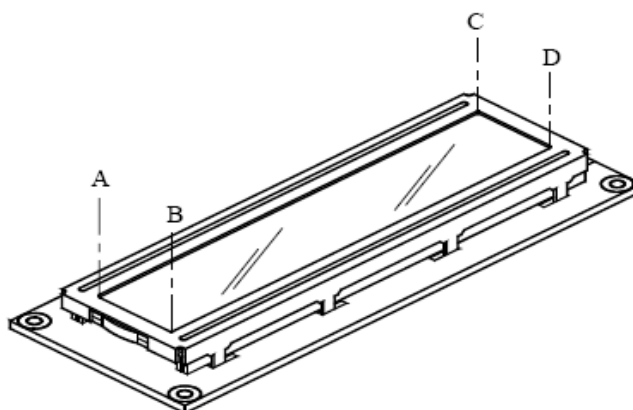
Direct Contact Discharge / Contact Point : A,B,C,D
