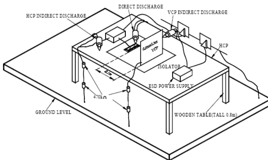
Direct Contact Discharge / Contact Point : A,B,C,D
