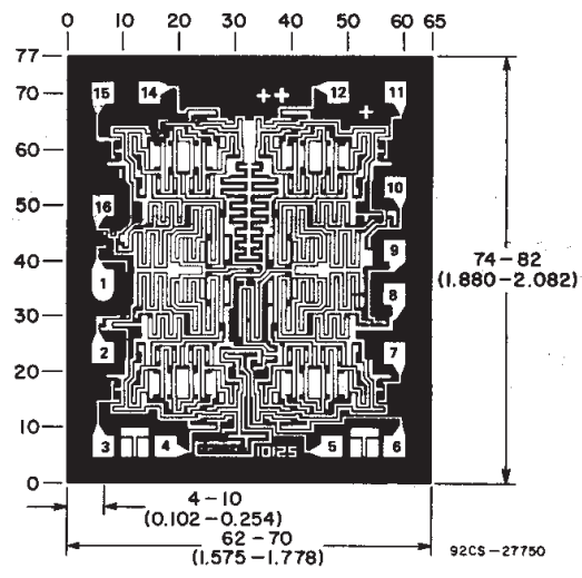
CD4043BH
